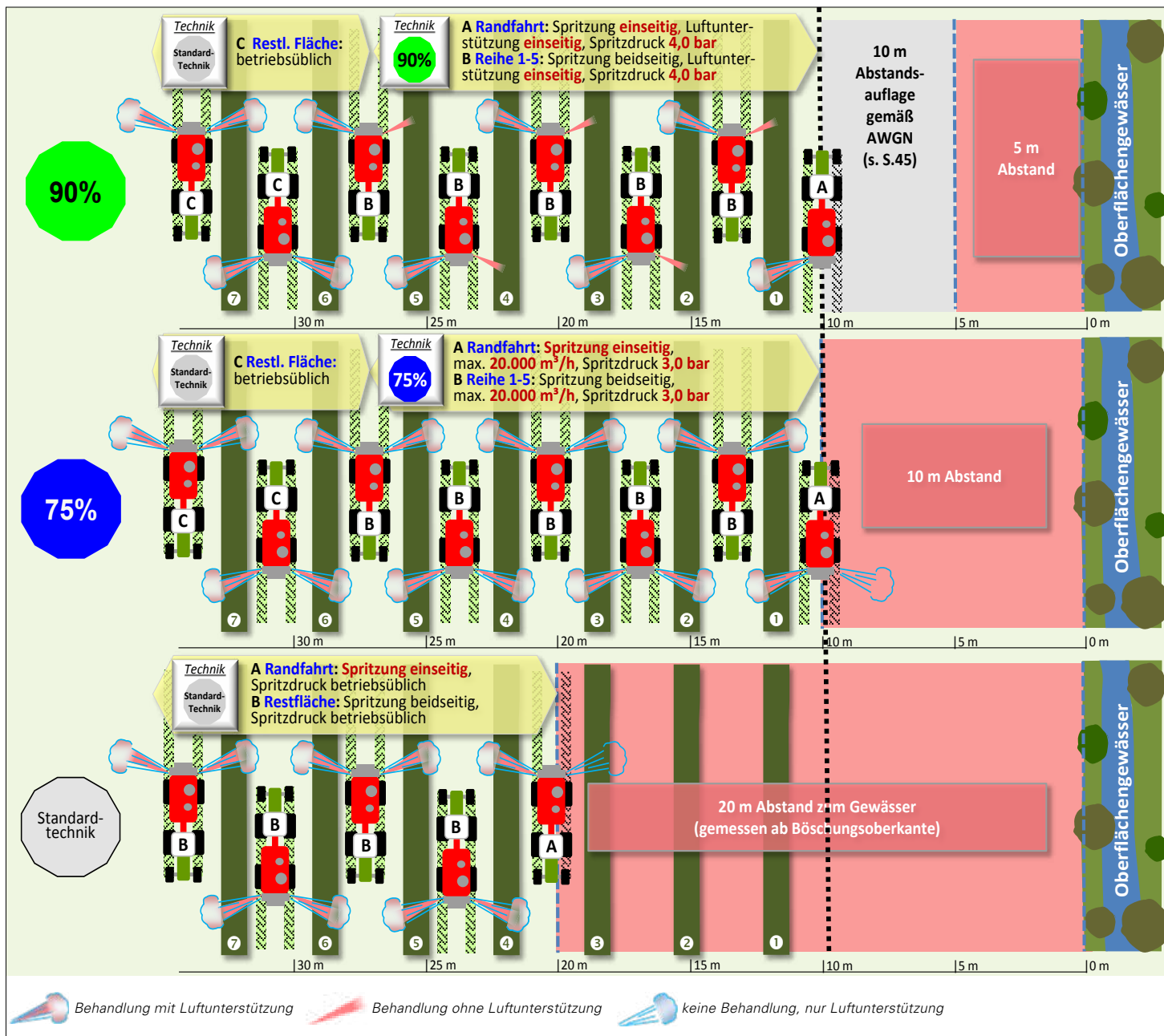
Schematische Darstellung der Abstandsauflagen zu Oberflächengewässern am Beispiel von Merpan 80 WDG in Kernobst
